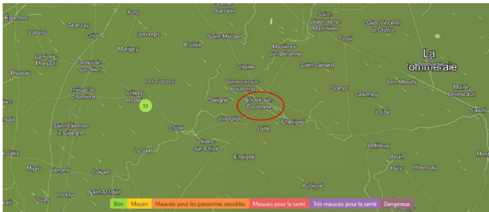
Figure 1 : Qualité de l'air à Brioux sur Boutonne
